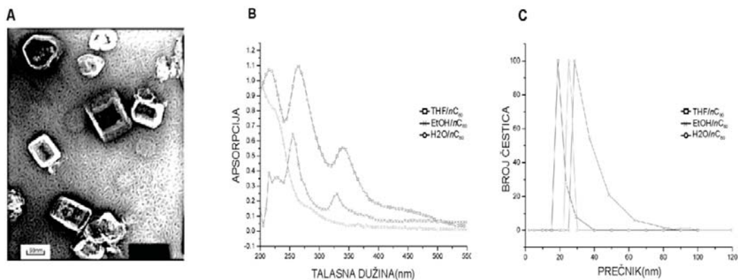
Slika 3. Karakterizacija fullerenskih koloida: (A) Fotografije nC_{60} kristala dobijene transmissionom elektronskom mikroskopijom. (B) UV-vis spektar apsorbanace različitih nC_{60} koloida. (C) Normalizovana distribucija veličinačestica različitih nC_{60} koloida.
