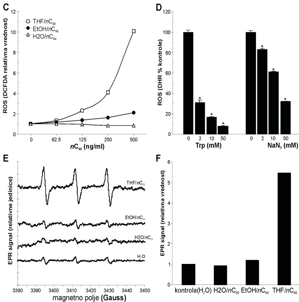
Slika 7. nC 60 čestice proizvode RKV u medijumu bez ćelija. (A) Promena fluorescencije DHR sa vremenom kao pokazatelj produkcije RKV u vodenom rastvoru nC 60 (0,5 μg/ml). (B, C) RKV produkcija zavisna od koncentracije različitih nC 60 u vodi (120 min) merena kao porast fluorescencije DHR (B) ili DCFDA (C). (D) Uticaj kvenčera singlet kiseonika (NaN 3 i triptofana-Trp) na proizvodnju RKV izazvanu THF/nC 60 nanočesticama (kontrola), merena kao fluorescencija DHR posle 120 minuta. (E, F) EPR merenje produkcije singlet kiseonika u rastvorima različitih nC 60 u poređenju sa kontrolnim uzorkom koji sadrži vodu. (A–F) Prikazani su rezultati reprezentativnog od najmanje tri izvedena eksperimenta. Podaci u (A–D) su srednje vrednosti triplikata (± SD u D; SD vrednosti u A–C su se kretale do 10% srednje vrednosti; *p < 0.05)
