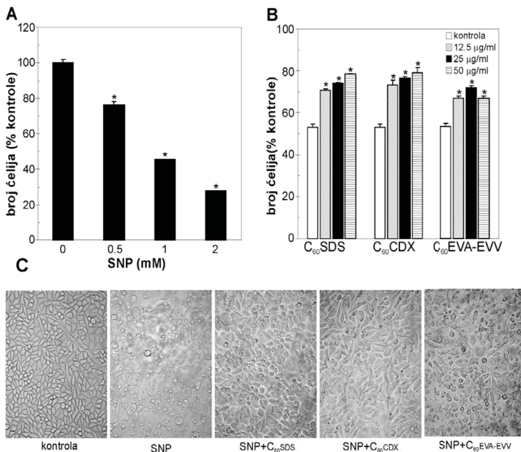
Slika 14. C 60 nanočestice smanjuju toksičnost NO. (A) L929 ćelije su 24 h inkubirane sa različitim koncentracijama NO donora SNP i broj ćelija je utvrđen kristal violet testom. (B, C) L929 ćelije su inkubirane sa SNP (1 mM) u prisustvu ili odsustvu različitih koncentracija (B) ili 50 µg/ml (C) C 60 nanočestica. Nakon 24 h je utvrđen broj ćelija kristal violet testom (B) ili je fazno-kontrastnim mikroskopom ispitana ćelijska morfologija (C). Podaci u (A, B) su predstavljeni kao srednja vrednost ± SD vrednosti triplikata iz reprezentativnog od tri nezavisna eksperimenta (*p < 0.05 je u odnosu na kontrole (A) ili ćelije tretirane SNP-om (B)).
