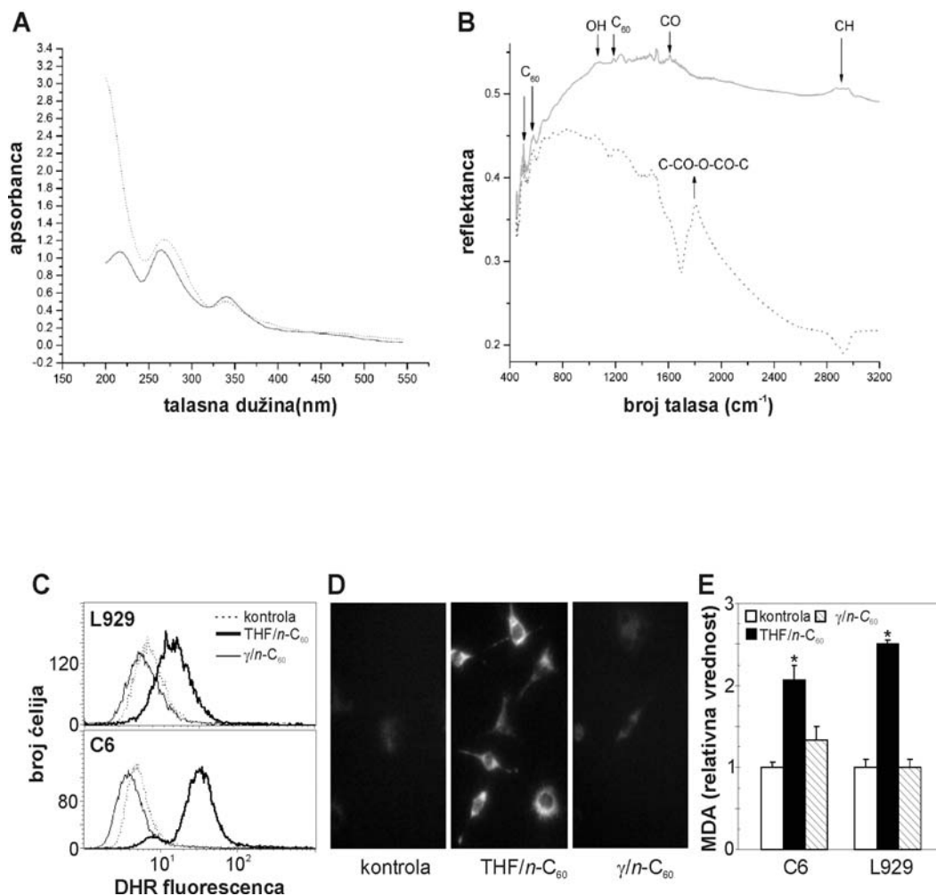
Slika 10. Gama zračenje blokira proizvodnju RKV izazvanu THF/nC 60 . Karakterizacija THF/nC 60 (puna linija) i γ/nC 60 (tačkasta linija) (A) UV-vis i (B) FTIR spektroskopskim analizama. Proizvodnja RKV je analizirana merenjem fluorescence DHR u C6 i L929 ćelijama tretiranim 3 h sa THF/nC 60 ili γ/nC 60 (1 μg/ml) i analiziranim (C) protočnom citofluorimetrijom ili (D) fluorescentnim mikroskopom u C6 ćelijama. (E) Malondialdehid (MDA), indikator lipidne peroksidacije, je meren u C6 i L929 ćelijama posle 6 h inkubacije sa 1 μg/ml THF/nC 60 ili γ/nC 60 . (E) Vrednosti su prikazane kao srednja vrednost ± SD triplikata iz reprezentativnog od najmanje tri eksperimenta (*p < 0.05 je u odnosu na kontrole i tretman sa ozračenim nC 60 ).
