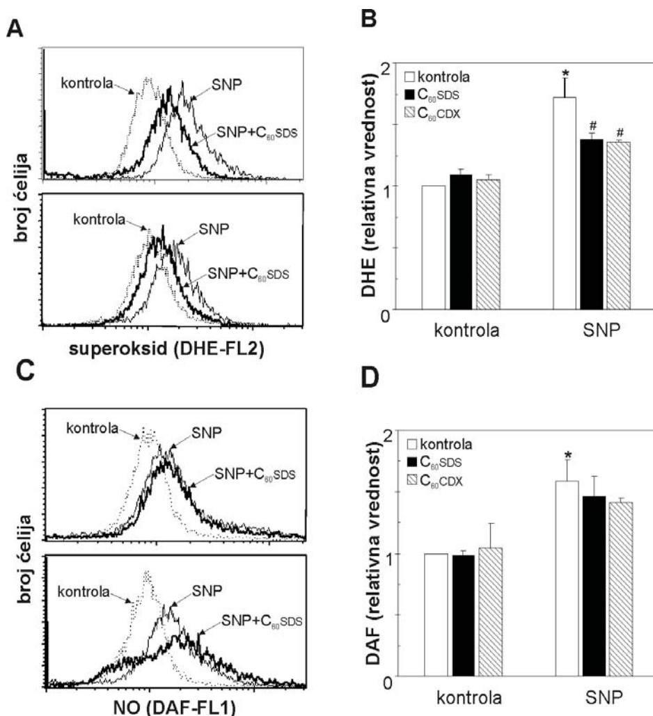
Slika 20. Uticaj C 60 nanočestica na proizvodnju superoksid anjona i NO u ćelijama tretiranim SNP-om. (A–D) L929 ćelije su inkubirane sa 1 mM SNP, u prisustvu ili odsustvu C 60 SDS ili C 60 CDX (50 μg/ml). Unutarćelijska produkcija superoksid anjona (A, B) i NO (C, D) je ispitana korišćenjem protočne citofluorimetrije u ćelijama obojenim odgovarajućim reporter bojama (DHE za O 2 - i DAF za NO). Prikazani su reprezentativni histogrami (A, C) dok su podaci u (B, D) srednje vrednosti ± SD iz tri eksperimenta (*p < 0.05 i #p < 0.05 su u odnosu na netretirane kontrolne ćelije ili ćelije tretirane SNP-om, respektivno).
