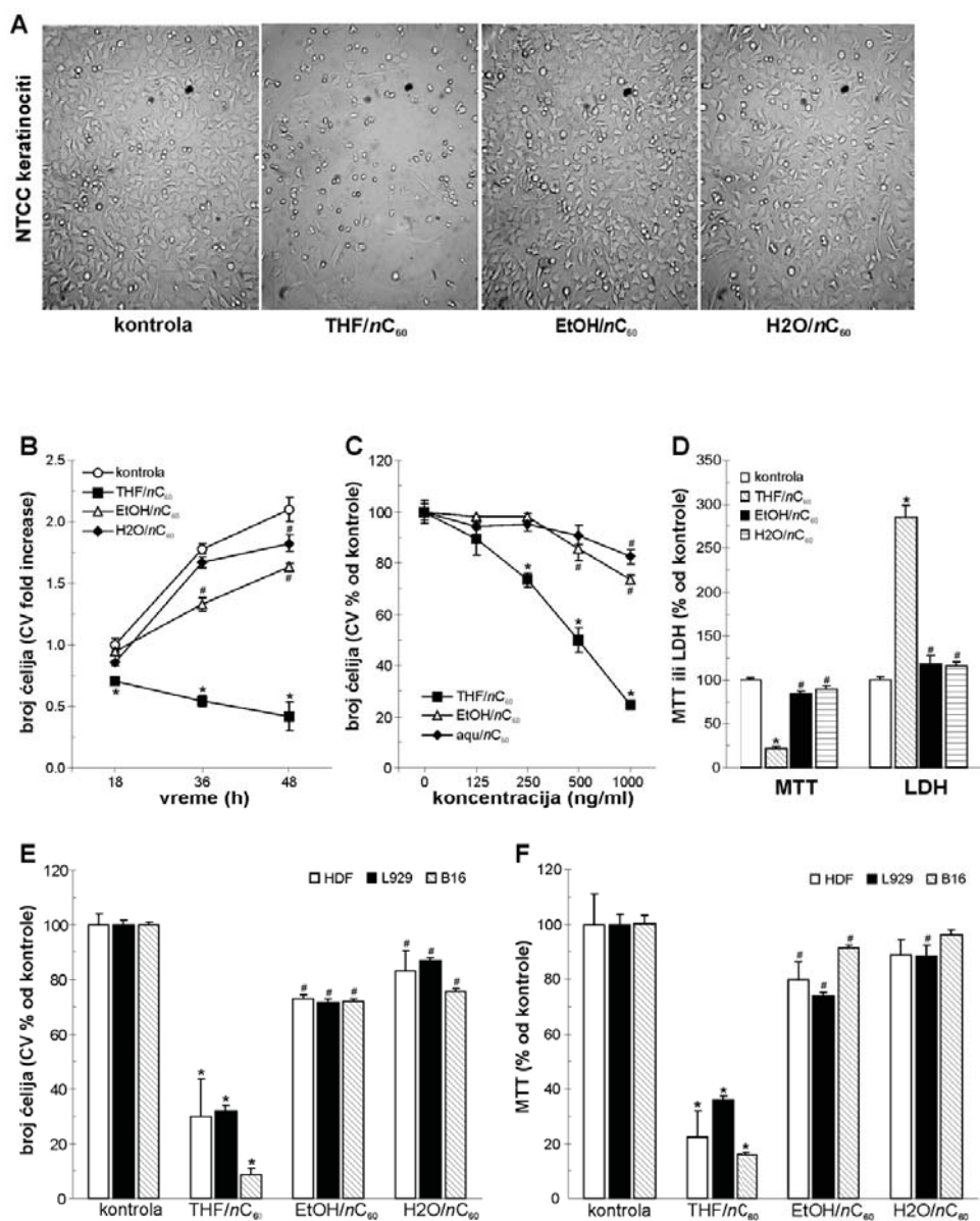
Slika 4 . Efekti različitih nC 60 koloida na ćelijsku morfologiju i vijabilitet. (A) NTCC ćelije tretirane rastvorima različitih nC 60 (1µg/ml, 48 h) posmatrane invertnim mikroskopom. (B) Vremenski zavisani uticaj različitih rastvora nC 60 (1µg/ml) na broj NTCC ćelija (kristal violet). (C) Promene u broju NTCC ćelija u zavisnosti od koncentracije različitih nC 60 koloidnih rastvora (mereno posle 48 h kristal violet testom). (D) Mitohondrijalna aktivnost (MTT) i oštećenje ćelijske membrane (LDH) kod NTCC ćelija koje su tretirane različitim rastvorima nC 60 (1µg/ml, posle 48 h). (E) Broj ćelija (kristal violet) i (F) mitohondrijalna aktivnost (MTT) kod HDF, L929 i B16 ćelijskih linija tretiranih sa različitim rastvorima nC 60 (1 µg/ml, posle 48 h). (B-F) Prikazani su reprezentativni rezultati iz najmanje tri eksperimenta kao srednja vrednost ± SD triplikata (* # p < 0.05 u odnosu na sve druge tretmane * ili na kontrolu # ).
