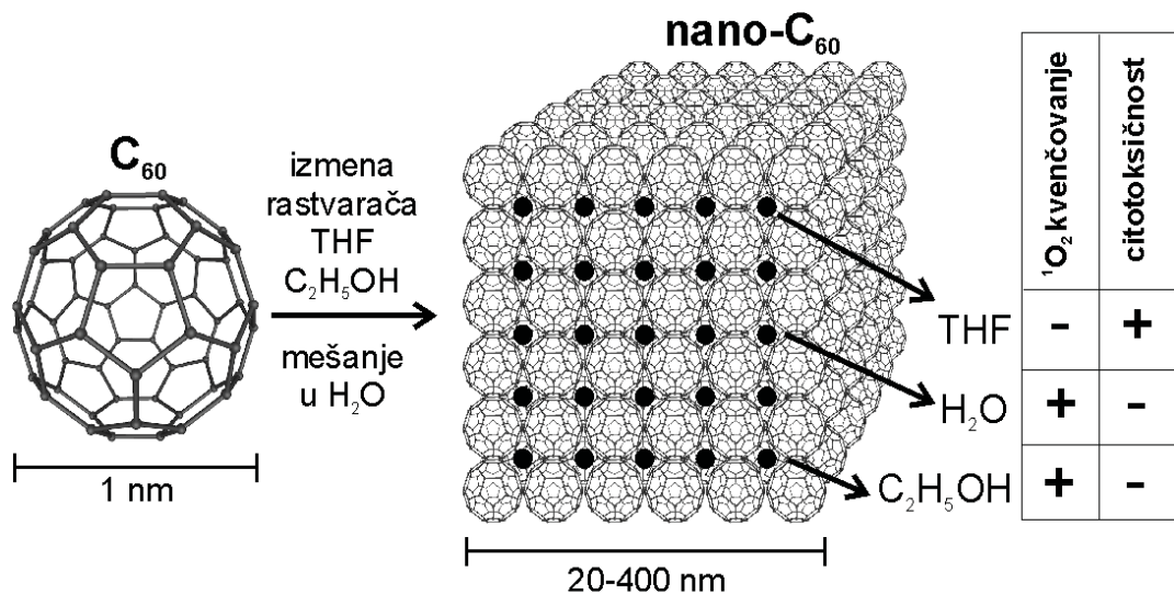
Slika 24. Shematski prikaz uticaja sposobnosti rastvarača da priguši ^1\text{O}_2 na citotoksičnost n\text{C}_{60} .
