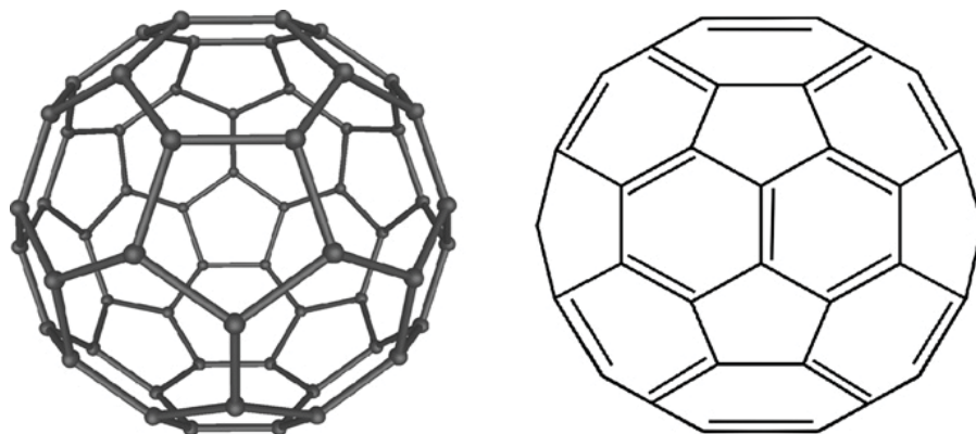
Slika 1. Struktura fullerena C_{60}
