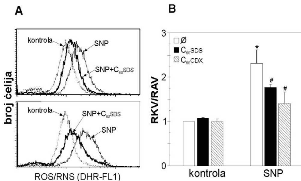
Slika 19. Uticaj C_{60} nanočestica na unutarćelijsku proizvodnju RKV i RAV. (A, B) L929 ćelije su inkubirane sa 1 mM SNP, sa ili bez 50 \mu g/ml C_{60}SDS ili C_{60}CDX . Unutarćelijska produkcija totalnog RKV/RAV je utvrđena protočnom citofluorimetrijom, korišćenjem DHR. Prikazani su reprezentativni histogrami, dok su rezultati (B) srednje vrednosti \pm SD iz tri odvojena eksperimenta (* p < 0.05 je u odnosu na netretirane kontrole, a # p < 0.05 na ćelije tretirane SNP-om)
