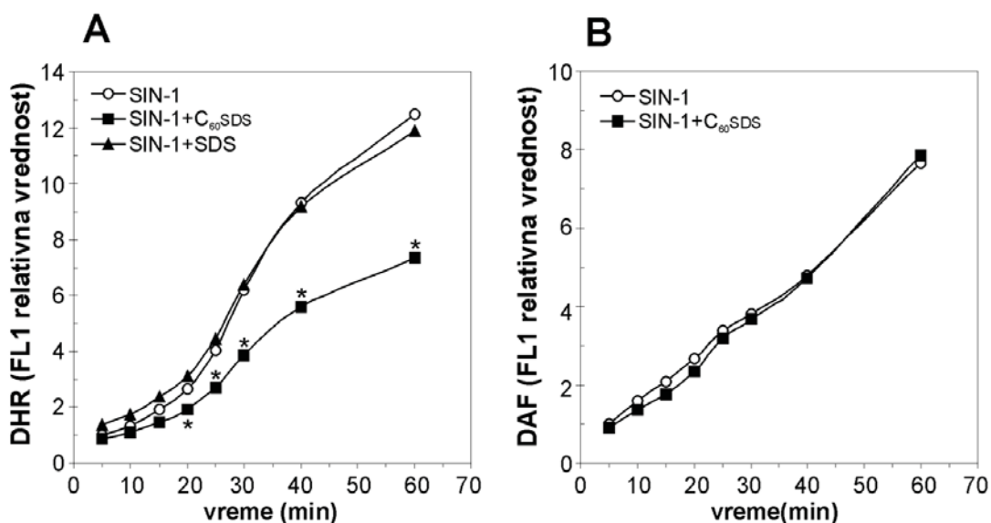
Slika 23. Efekti C_{60} nanočestica na produkciju RKV i RAV u rastvoru SIN-1. (A, B) NO/superoksid donor SIN-1 (0.2 mM) je rastvoren u fosfatnom puferu, sa ili bez 50 \mu g/ml C_{60} SDS (A, B) ili 6.25 \mu g/ml SDS (A). DHR i DAF fluorescencija je merena u određenim vremenskim intervalima. Dobijeni podaci su srednje vrednosti \pm SD triplikata iz reprezentativnog od tri eksperimenta (* p < 0.05 ; SD vrednosti su bile < 5\% od srednje vrednosti).
