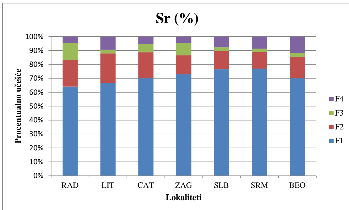
Grafik 52. – Raspedela Sr po fazama sekvencijalne ekstrakcije (I, II, III, i IV faza) u uzorcima sedimenta iz 2014. godine
