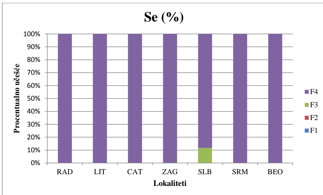
Grafik 51. – Raspedela Se po fazama sekvencijalne ekstrakcije (I, II, III, i IV faza) u uzorcima sedimenta iz 2014. godine
