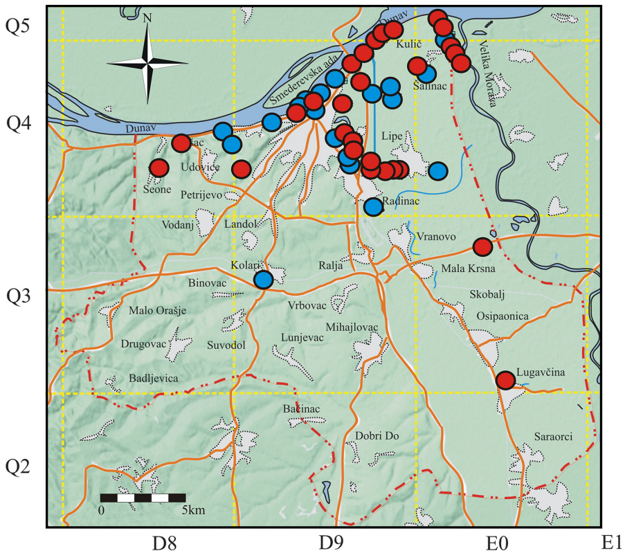
Fig. 10. – Distribution of Pelophylax kl. esculentus (Linnaeus, 1758) in Smederevo municipality.
