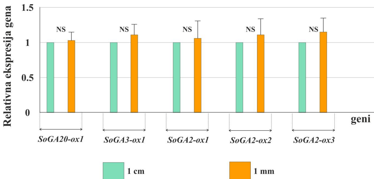
Slika 23. Ekspresija SoGA20-ox1 , SoGA3-ox1 , SoGA2-ox1 , SoGA2-ox2 i SoGA2-ox3 u apikalnim odsečcima korenova veličine 1 cm ili 1 mm. Eksplantati su izolovani sa 15 nasumično odabranih klijanaca iz populacije, nakon čega su zamrznuti u tečnom azotu. Kao kalibrator su korišćeni eksplantati veličine 1 cm. Ekspresija je normalizovana u odnosu na ekspresiju gena za \alpha -tubulin upotrebom \Delta\Delta C_t metoda. Podaci predstavljaju srednje vrednosti \pm standardna greška tri biološka ponavljanja, svako sa tri tehnička ponavljanja. Statistička značajnost je određena t-testom za zavisne uzorke. NS - nema statistički značajnih razlika.
