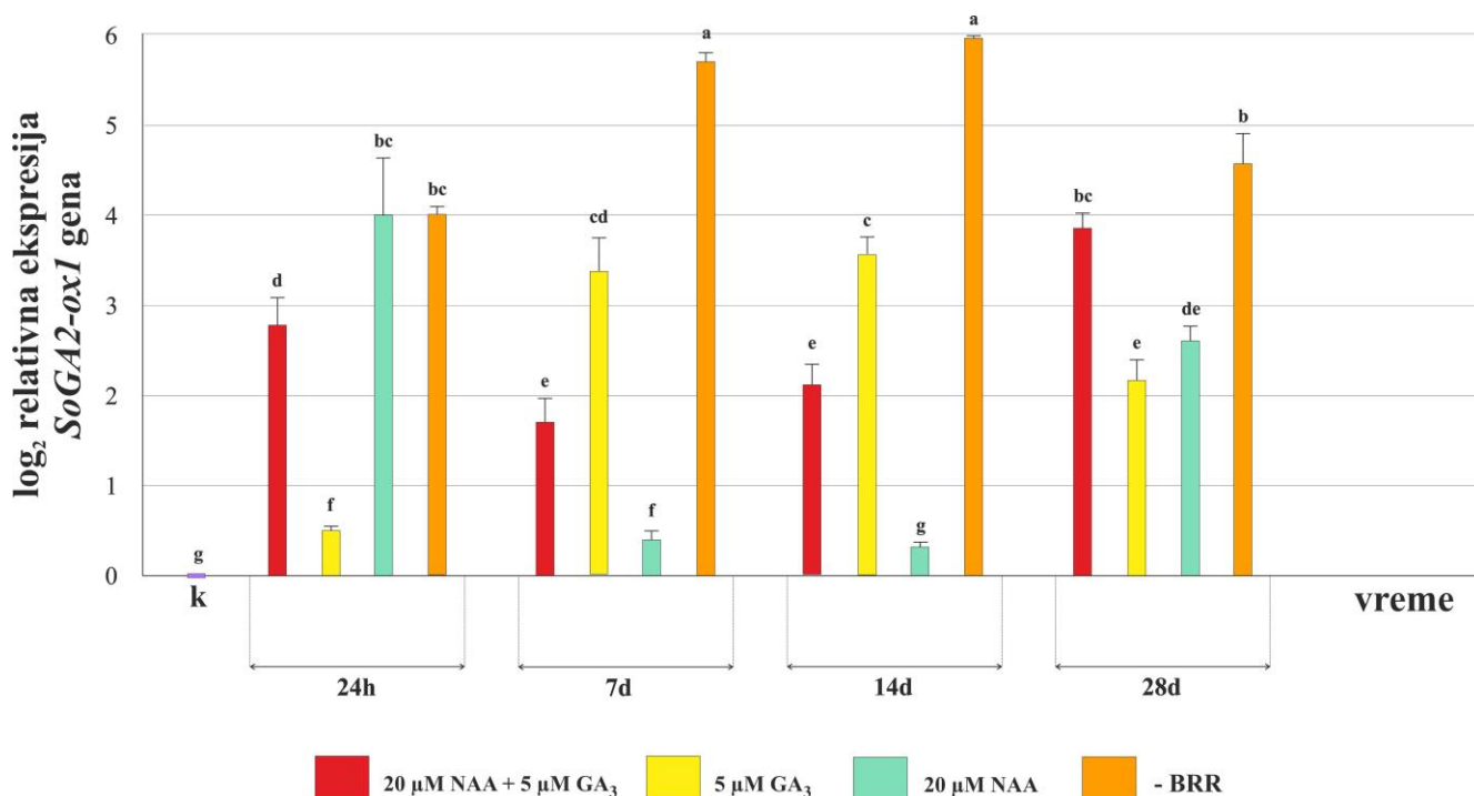
Slika 27. Ekspresija SoGA2-ox1 u apikalnim odsečcima korenova kultivisanim tokom 1, 7, 14 ili 28 dana na IMSE (20 \mu\text{M} NAA + 5 \mu\text{M} GA 3 ), medijumu bez BRR ili na medijumu koji je sadržao 5 \mu\text{M} GA 3 ili 20 \mu\text{M} NAA. Kao kalibrator su korišćeni eksplantati koji su odmah po izolaciji sa klijanaca zaleđeni u tečnom azotu. Ekspresija je normalizovana u odnosu na ekspresiju gena za \alpha -tubulin upotrebom \Delta\Delta\text{C}_t metoda. Podaci predstavljaju srednje vrednosti \pm standardna greška tri biološka ponavljanja, svako sa tri tehnička ponavljanja. Vrednosti na grafiku označene istim slovima nisu statistički značajno različite ( p \leq 0.05 ) prema LSD testu.
