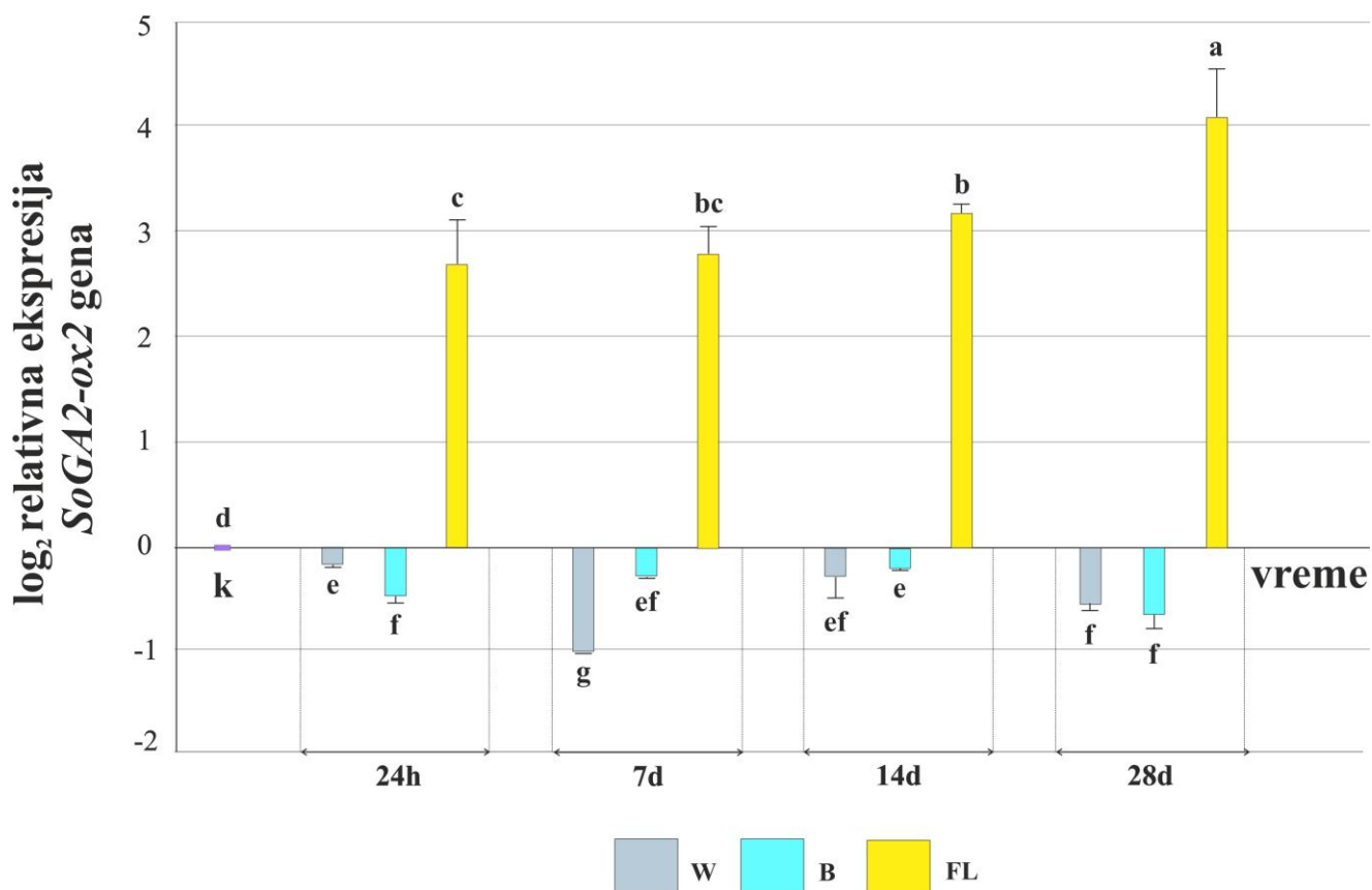
Slika 40. Ekspresija SoGA2ox-2 u apikalnim odsečcima korenova gajenim gajenih na IMSE pod uticajem FL (380-680 nm, 17 \mu\text{mol m}^{-2}\text{s}^{-1} ) i LED osvetljenja iz oblasti B dela spektra (460 nm, 10.5 \mu\text{mol m}^{-2}\text{s}^{-1} ) i W spektra ( 16 \mu\text{mol m}^{-2}\text{s}^{-1} ). Ekspresija je normalizovana u odnosu na ekspresiju gena za \alpha -tubulin. Kao kalibrator su korišćeni eksplantati koji su odmah po izolaciji sa klijanaca zaleđeni u tečnom azotu. Podaci predstavljaju srednje vrednosti \pm standardna greška tri biološka ponavljanja, svako sa tri tehnička ponavljanja. Vrednosti na grafiku označene istim slovima nisu statistički značajno različite ( p \leq 0.05 ) prema LSD testu.
