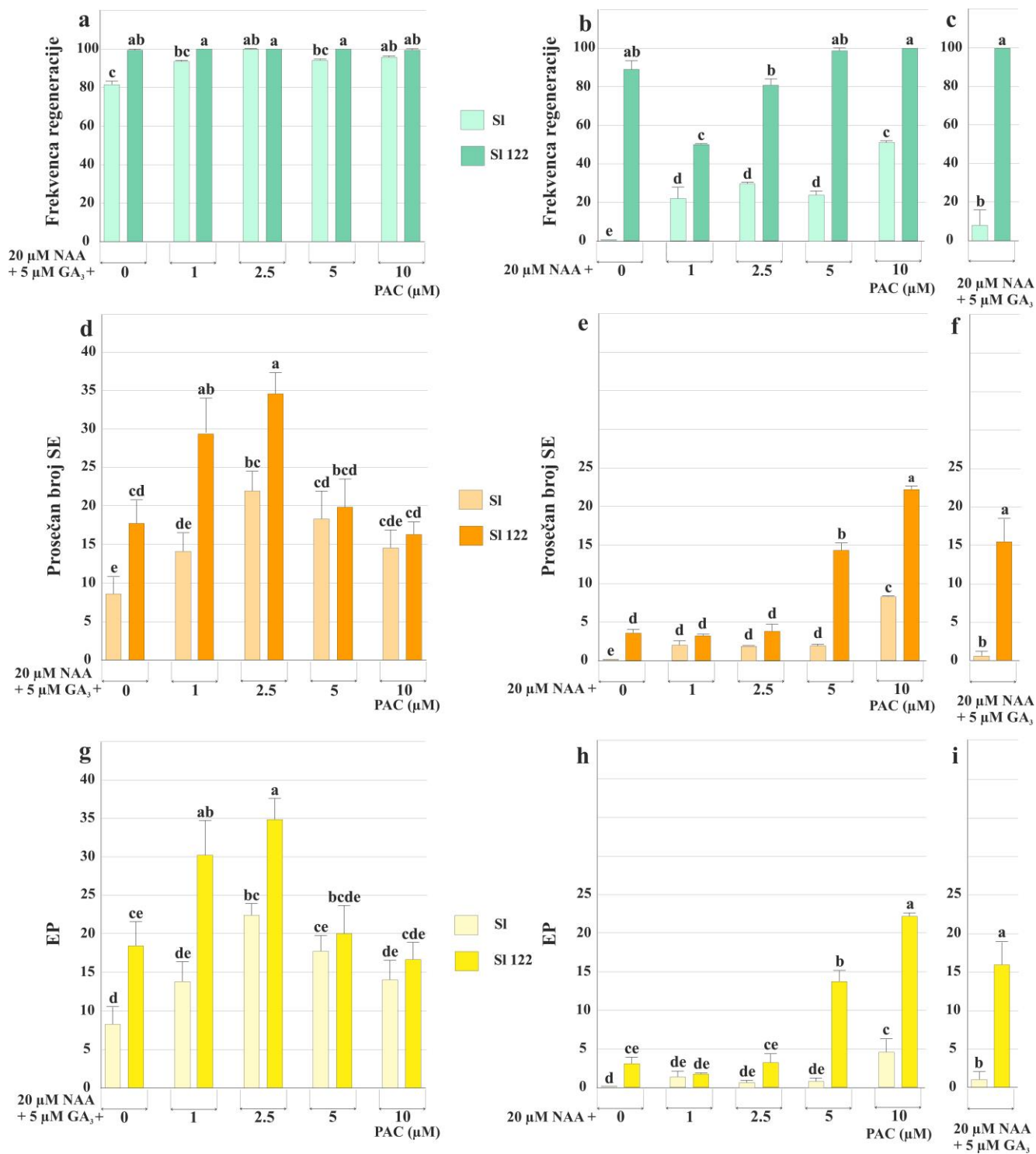
Slika 16. Uticaj PAC na embriogeni potencijal apikalnih odsečaka korenova spanaća. Eksplantati su gajeni na IMSE (20 μM NAA + 5 μM GA 3 ) uz dodatak 0-10 μM PAC ( a, d, g ) ili na medijumu koji je sadržao 20 μM NAA uz dodatak 0-10 μM PAC ( b, e, h ) tokom 12 nedelja. Za testiranje punog embriogenog potencijala grupe klijanaca kultivisanih na 20 μM NAA + 0-10 μM PAC, postavljena je kontrola genetički identičnog materijala kultivisanog na IMSE bez PAC ( c, f, i ). ( a, b, c ) Frekvencija regeneracije. ( d, e, f ) Prosečan broj SE. ( g, h, i ) EP indeks. Podaci predstavljaju srednje vrednosti ± standardna greška. Za svaki tretman su postavljene tri petri kutije sa po 10-15 eksplantata (n=30-45). Vrednosti na grafiku označene istim slovima nisu statistički značajno različite (p≤0.05) prema LSD testu.
